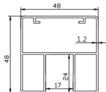
尺寸展示
