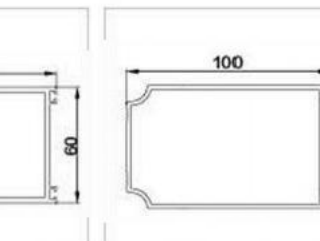
型号: GM-608A 名称: 灯带主梁 重量: 3.194kg/m 壁厚: 2.8mm
