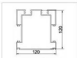
型号: GM-604 名称: 120立柱 重量: 4.228kg/m 壁厚: 3.0mm
