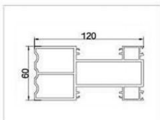
型号: GM-602 名称: 120g 重量: 3.31kg/m 壁厚: 3.0mm
