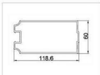
型号: GM-6082.0 名称: 120主梁 重量: 1.963kg/m 壁厚: 2.0mm
