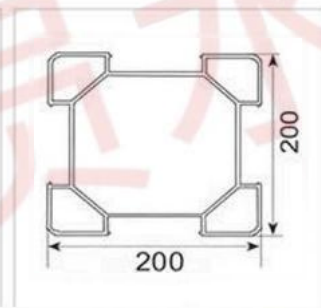
型号: GM-168-218 名称: 200罗马柱 重量: 10.83kg/m 壁厚: 3.5mm
