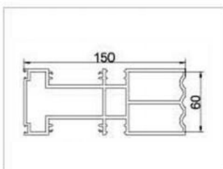
型号: GM-603 名称: 150梁 重量: 4.412kg/m 壁厚: 3.0mm
