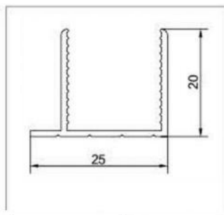
型号: PT-60 名称: 扣板外F槽 重量: 0.18kg/m 壁厚: 1.0mm
