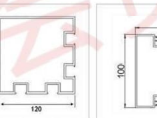
型号: GM-168-284 名称: 120立柱 重量: 4.68kg/m 壁厚: 3.0mm
