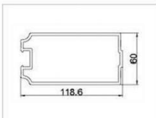
型号: GM-6083.0 名称: 120主梁 重量: 2.818kg/m 壁厚: 2.9mm
