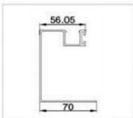
型号: GM-621 名称: 拼装水槽 重量: 1.207kg/m 壁厚: 1.6mm
