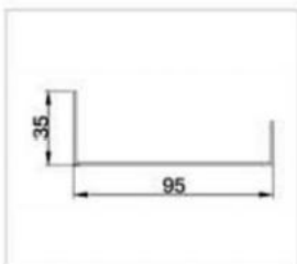
型号: GM-952 名称: 装饰板 重量: 0.482kg/m 壁厚: 1.2mm
