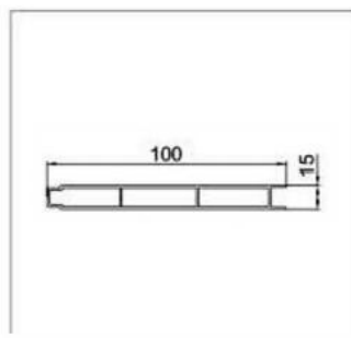
型号: PT-61 名称: 罗马柱扣板 重量: 0.79kg/m 壁厚: 1.1mm
