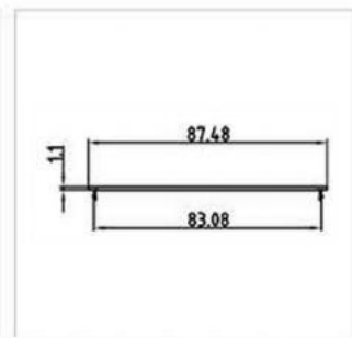
型号: GM-168-220 名称: 罗马柱盖板 重量: 0.32kg/m 壁厚: 1.1mm
