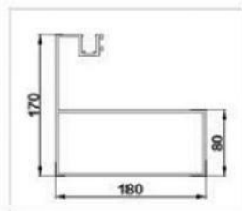
型号: GM-614 名称: 边框水槽 重量: 8.63kg/m 壁厚: 2.9mm
