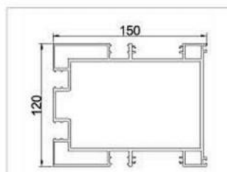
型号: GM-605 名称: 150立柱 重量: 5.34kg/m 壁厚: 3.0mm
