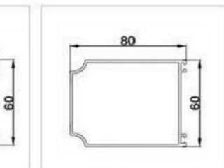
型号: GM-616 名称: 100主梁 重量: 1.69kg/m 壁厚: 2.0mm
