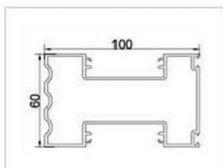
型号: GM-606 名称: 100梁 重量: 1.88kg/m 壁厚: 2.0mm
