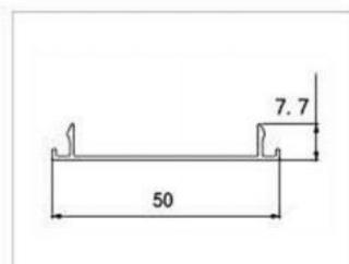
号: PT-20 名称: 开口管座椅盖子 重量: 0.167kg/m 壁厚: 0.9mm
