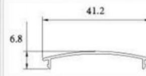
型号: FS-25B 名称: 压盖 重量: 0.118kg/m 量厚: 0.9mm
