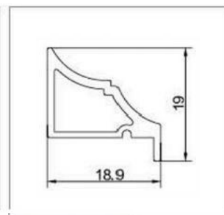
型号: PT-26 名称: 120罗马柱装饰线 重量: 0.20kg/m 壁厚: 1.2mm
