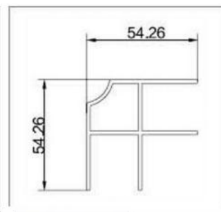
型号: PT-63 名称: 罗马柱扣条 重量: 0.44kg/m 壁厚: 1.2mm
