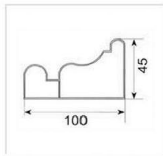
型号: GM-168-118 名称: 100罗马柱 重量: 0.9kg/m 壁厚: 1.2mm
