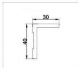
型号: GM-951 名称: 传动条 重量: 0.167kg/m 壁厚: 4.0mm
