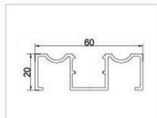
型号: GM-612 名称: 附加料 重量: 0.616kg/m 壁厚: 2.0mm
