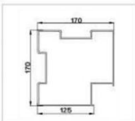
型号: GM-617 名称: 170罗马立柱 重量: 5.12kg/m 壁厚: 2.5mm
