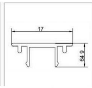
型号: PT-03 名称: 四角小压线 重量: 0.073kg/m 壁厚: 1.0mm
