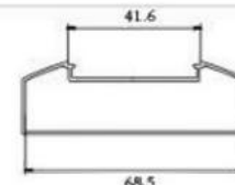
型号: FS-25A 名称: 盟管 重量: 0.505kg/m 壁厚: 1.0mm
