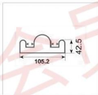
型号: PT-09 名称: GM-LG0149 重量: 0.692kg/m 壁厚: 1.4mm
