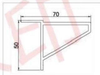
型号: GM-611 名称: 转换梁 重量: 1.18kg/m 壁厚: 2.5mm
