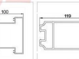
型号: GM-613 名称: 100边梁 重量: 2.565kg/m 壁厚: 2.0mm
