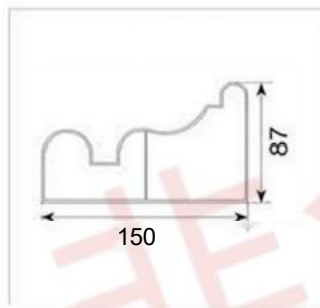
型号: GM-168-263 名称: 150罗马柱 重量: 2.3kg/m 壁厚: 1.4mm
