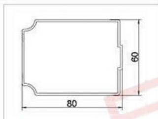
型号: GM-609 名称: 80副梁 重量: 1.14kg/m 壁厚: 2.0mm
