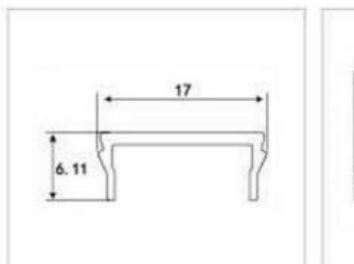
型号: GM-168-232 名称: 120靠墙压普 重量: 0.073kg/m 壁厚: 1.0mm
