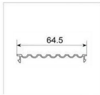
型号: PT-28 名称: 100罗马柱盖帽 重量: 0.22kg/m 壁厚: 0.3mm
