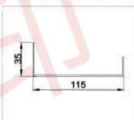
型号: 名称: 装饰板 重量: 0.5kg/m 壁厚: 1.2mm
