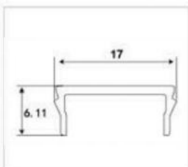
型号: GM-168-232 名称: 120阳光房压板 重量: 0.073kg/m 壁厚: 1.0mm
