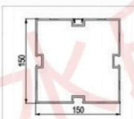
型号: 150*150 名称: 罗马立柱 重量: 4.512kg/m 壁厚: 2.5mm
