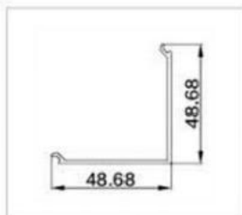
型号: GM-619 名称: 1708柱装饰 重量: 0.358kg/m 壁厚: 1.3mm
