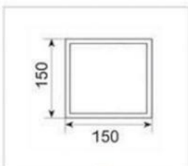
型号: PT-10 名称: 大方管 重量: 4.8kg/m 壁厚: 3.0mm
