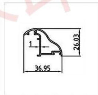
型号: GM-168-219 名称: 罗马柱装饰线 重量: 0.316kg/m 壁厚: 1.0mm
