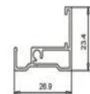
名称: 外框料 型号: JSF-1647 壁厚: 0.9 米重: 0.24
