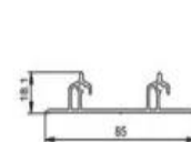
名称: 至尊1双下轨 型号: JSF-1445 壁厚: 1.2 米重: 0.566
