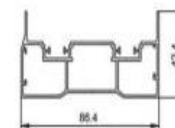
名称: 堆尚4号边封 型号: JSF-1605 壁厚: 1.2 米重: 1.12
