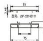
名称: 75平盖中横 型号: JSF-20180111 壁厚: 1.0 米重: 0.7
