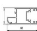
名称: 80 扇门扇玉 型号: JSF-1606 壁厚: 1.3 米重: 1.1
