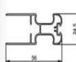
名称: 拉杆 型号: JSF-2116 壁厚: 0.8 米重: 0.48
