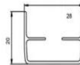
22款2.0网折铝材 型号: JSF-2204 壁厚: 1.0 米重: 0.217
