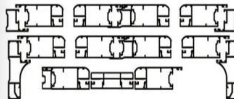
名称: 中横 型号: JSF-2017013 壁厚: 0.9 米重: 0.54
