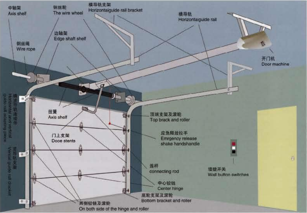
车库门安装示意图
